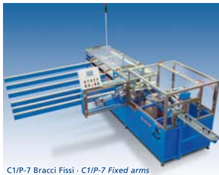
C1/P-7 Bracci Fissi · C1/P-7 Fixed arms
