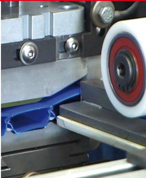
Dettaglio dell'avvolgibile durante il confezionamento Detail of the roller shutter during the assembly phase
